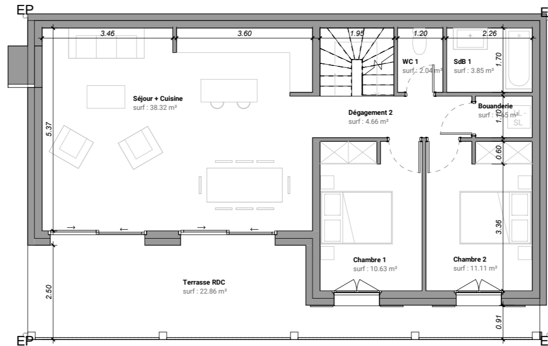
PLAN RDC
